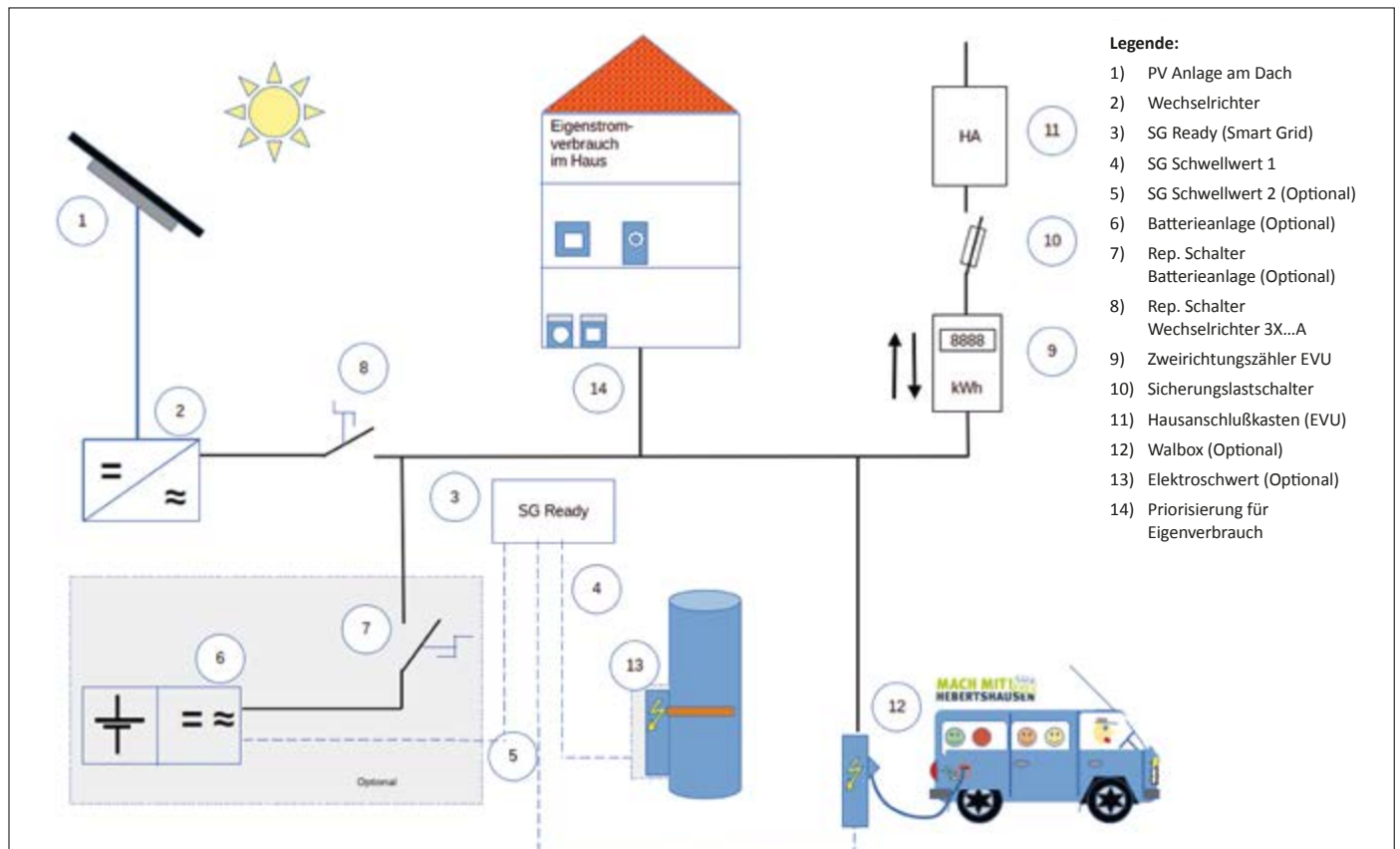
Darstellung der wichtigsten Komponenten einer Photovoltaikanlage.
